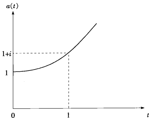
图 1-1 累积函数
