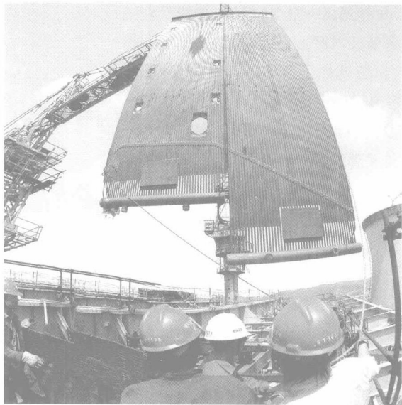
2003年以来,我省相继建设一批60万千瓦及以上的超临界、超超临界燃煤脱硫机组。截至2007年底,全省6000千瓦及以上发电装机4328万千瓦,是1978年162万千瓦的27倍。图为浙江新能兰溪发电公司60万千瓦超临界发电机组的锅炉在安装。
