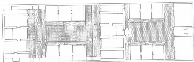
图 611-10 总平面 宋昆《平遥古城与民居》
