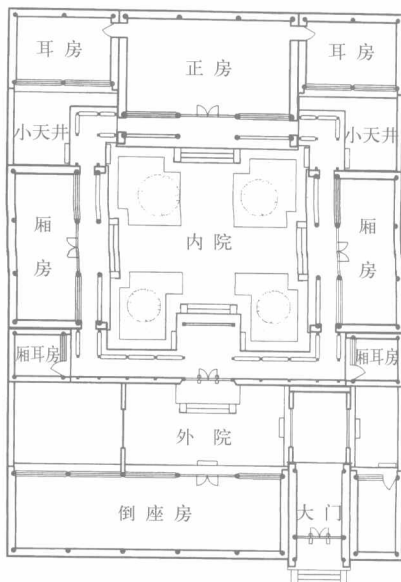
图 611-4 四合院平面中的躲闪关系 马炳坚《北京四合院建筑》
