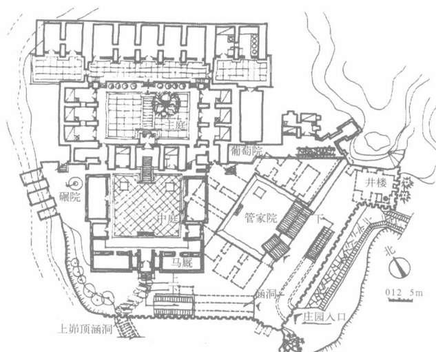
图 611-17 米脂县刘家峁姜园总平面 侯幼彬《中国古代建筑历史图说》
