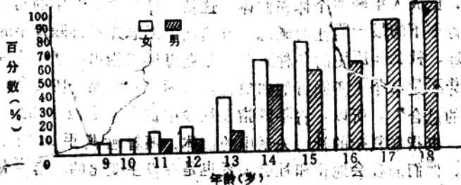
图 1—1 性成熟过程的性别差异
