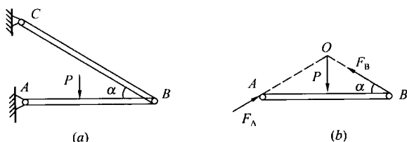
图 9-3 三力平衡必汇交
