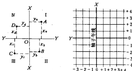
图 1-5 测量计算的平面直角坐标系
