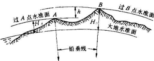
图 1-6 点的高程
