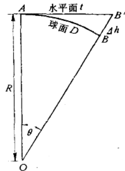
图 1-7 地球曲率的影响
