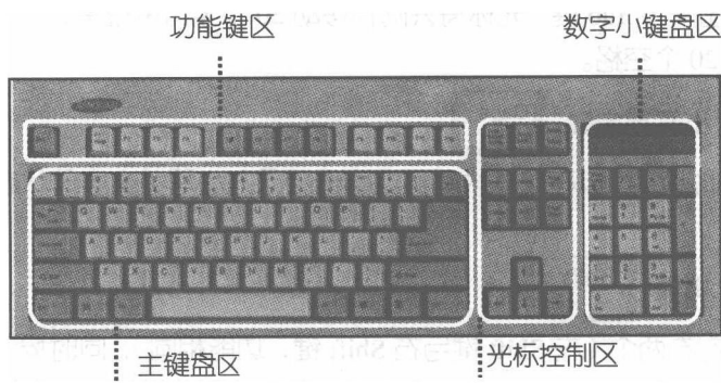
图 1-4 键盘分区图
