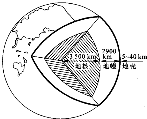
图 1-1 地球的内部分层
