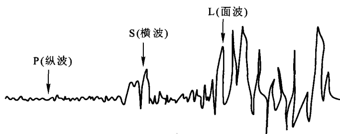
图 1-5 地震波记录示意图
