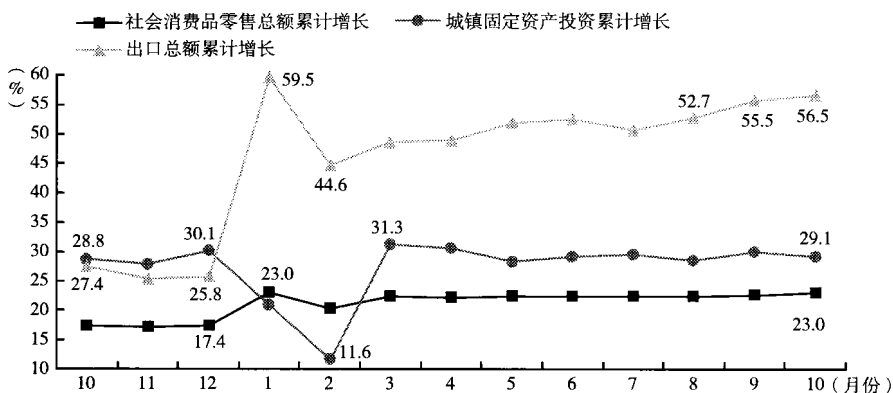
图2 投资、消费和出口总额累计增长
