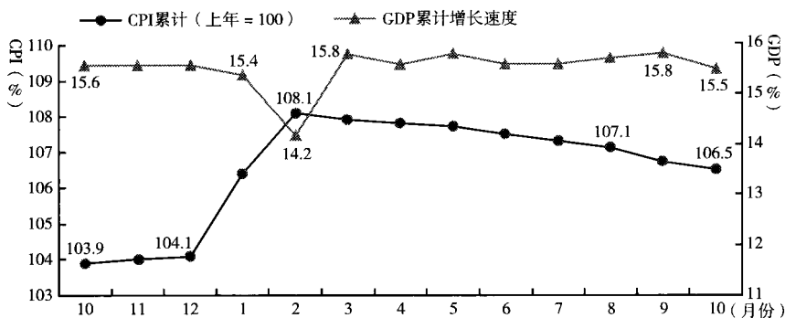
图1 GDP 累计增长和 CPI 累计
