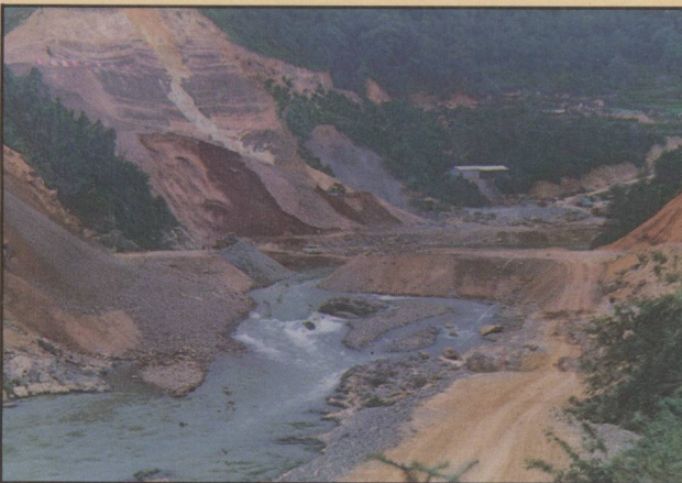
雙溪水電站工程，總投資 3.12 億元，裝機容量 3.6 萬千瓦，由中國水利水電長江葛洲壩工程局承建。左圖為即將合攏的電站大壩。右圖為開鑿電站隧道工地
