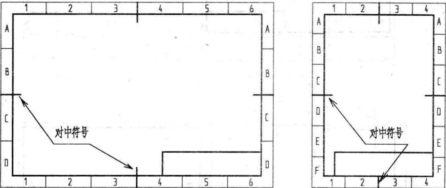
图 1-5 图幅分区和对中符号
