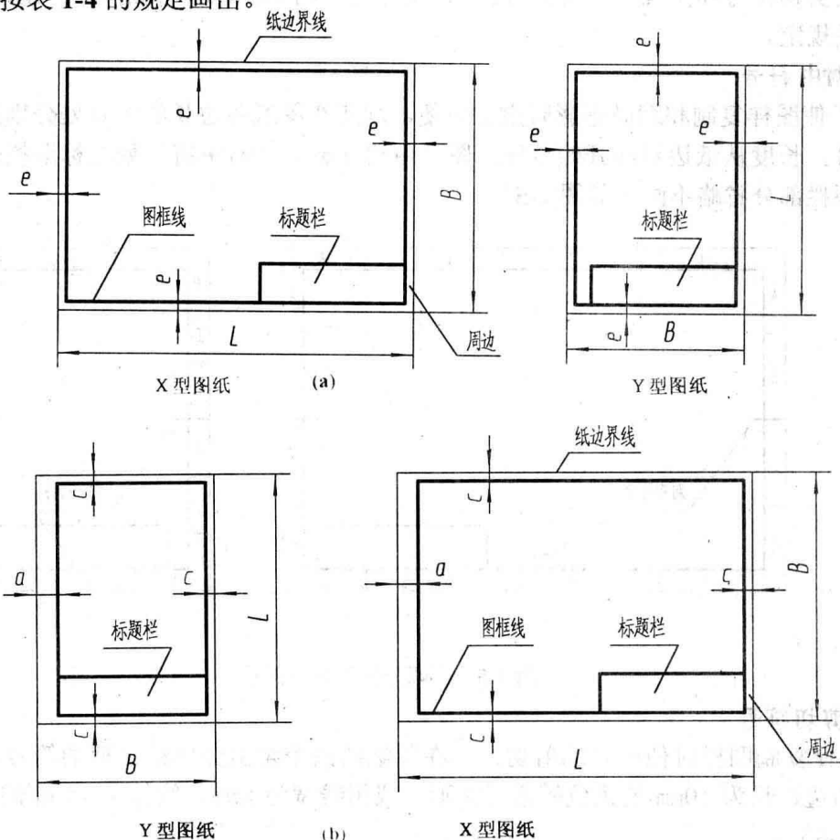
图 1-3 图框格式
