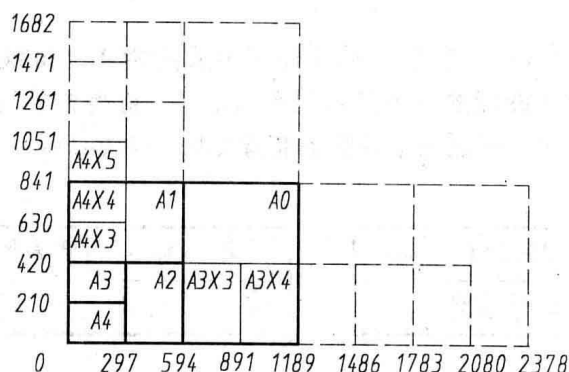
图 1-2 图纸幅面
