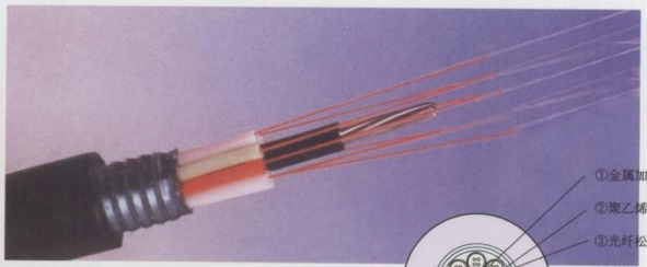
光缆结构
