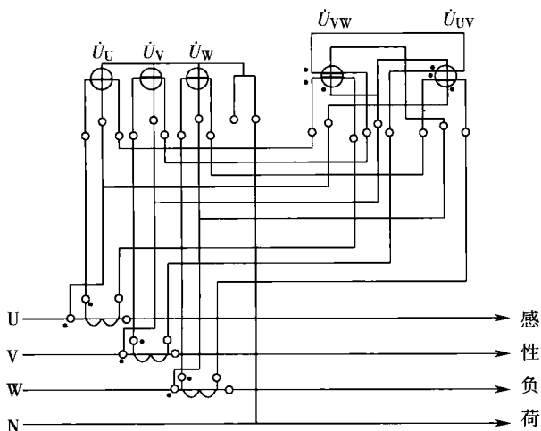
图 1-3 三相四线高供低计电能计量装置的接线图
