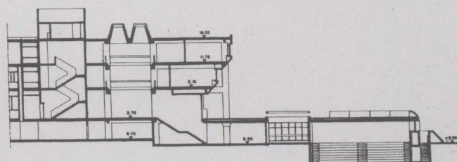
剖面 IV
