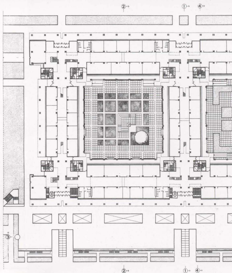
一层平面图
