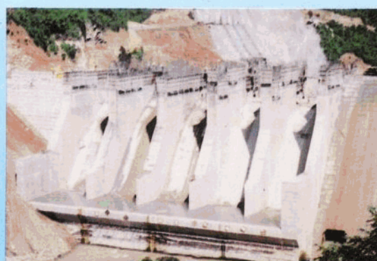
采用国际最新施工技术全断面混凝土碾压坝的双溪水电站(水库)大坝
