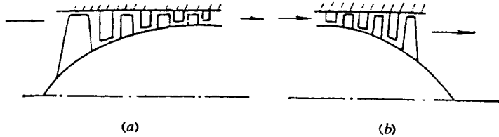
图 1-1 轴流式叶片机示意图
