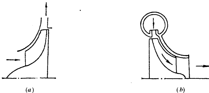
图 1-2 径流式叶片机示意图
