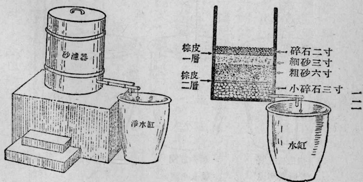
第七圖 砂濾法
