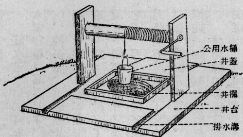
第一圖 水井的改良 (井欄方形、圓形皆可)
