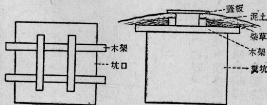
第八圖 深坑小口廁所
