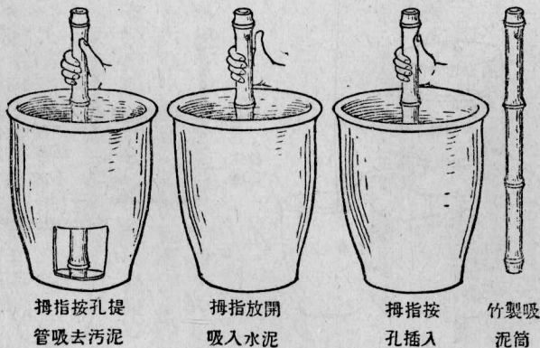
第六圖 吸泥筒使用法
