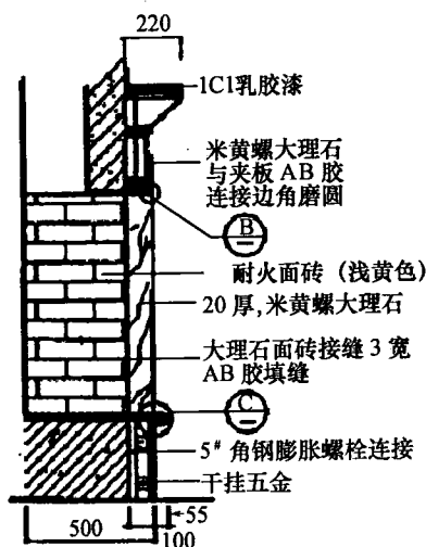
剖面图
