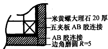
ⓑ 节点详图
