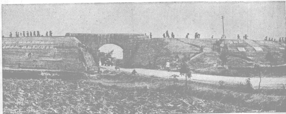
长寿县东风大堰，流灌石堰、双龙、葛兰等三个人民公社，干渠全长九十四公里。
