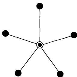
图 1.7 K_{1,5}
