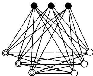
图 1.8 K_{3(3)}
