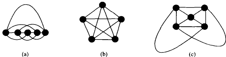
图 1.5 K_5
