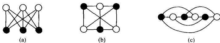
图 1.6 K_{3,3}
