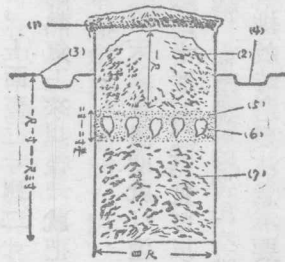
（二）寬方向縱剖面圖
