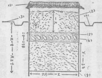
（一）長方向縱剖面圖
