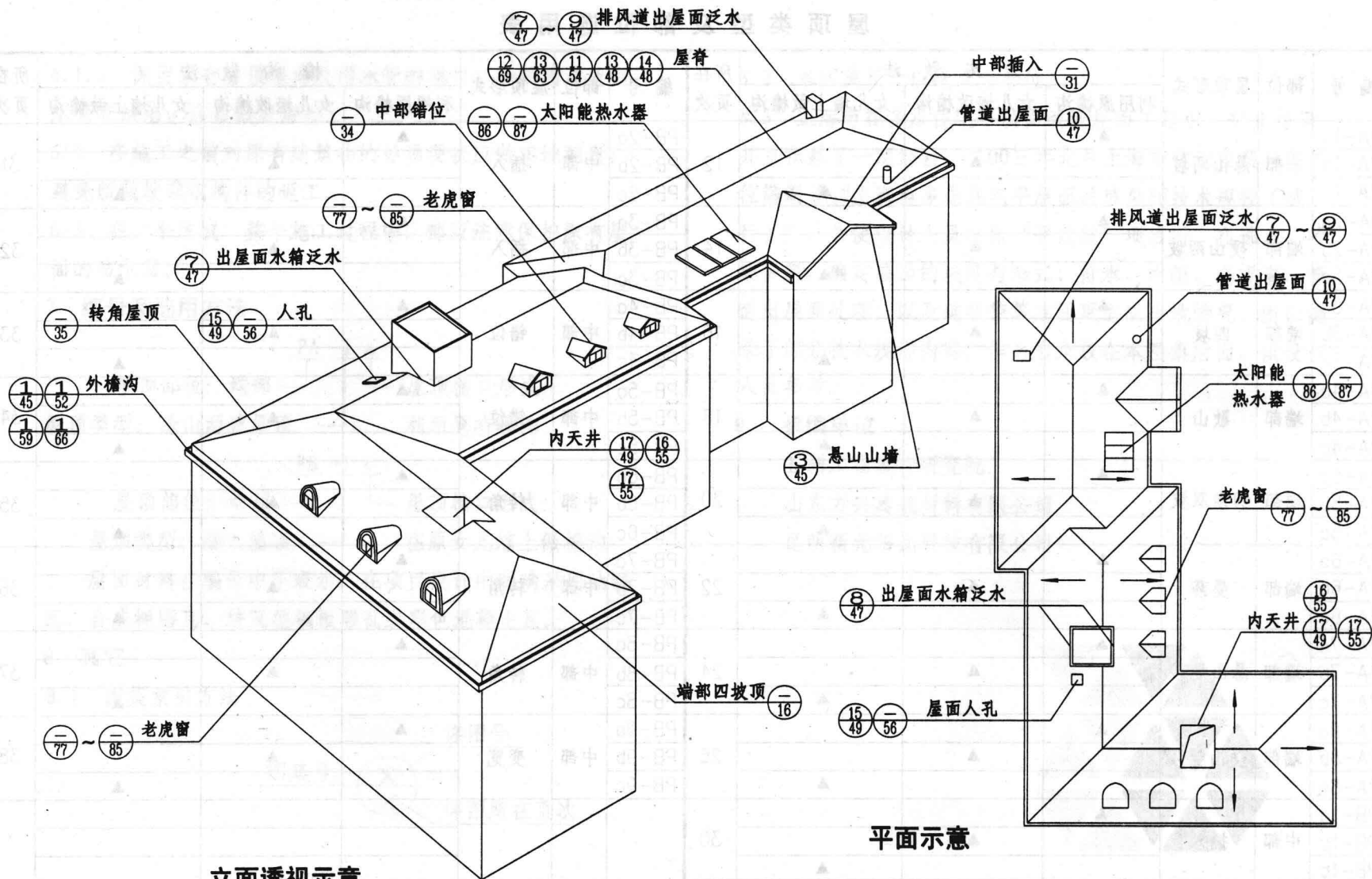
立面透视示意
