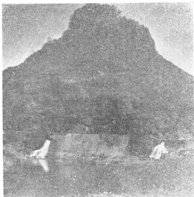
宜山县里洞水库地下河出口堵体
