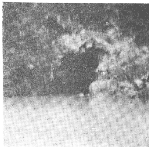
钟山县川岩地下河出口
