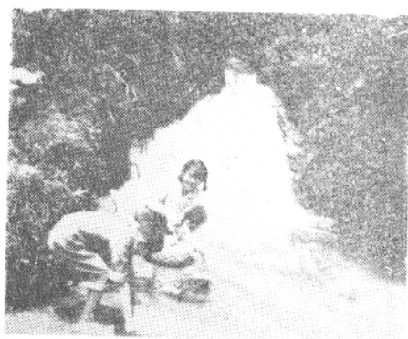
隆林县蛇场公社一下降泉
