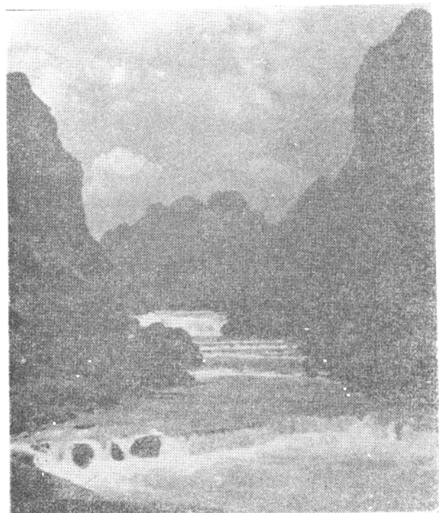
大新县黑水河中上游多级跌水
