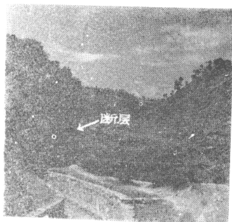
隆安县布良水库二级洼地末端垭口断层
