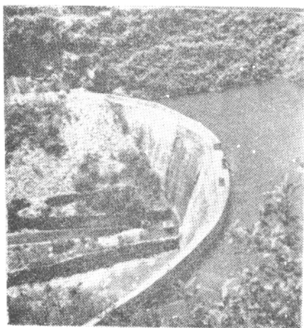
隆林县蛇场公社斗峰坡水库坝首
