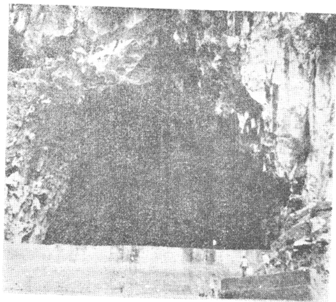
上林县大龙洞水库溢洪洞进口
