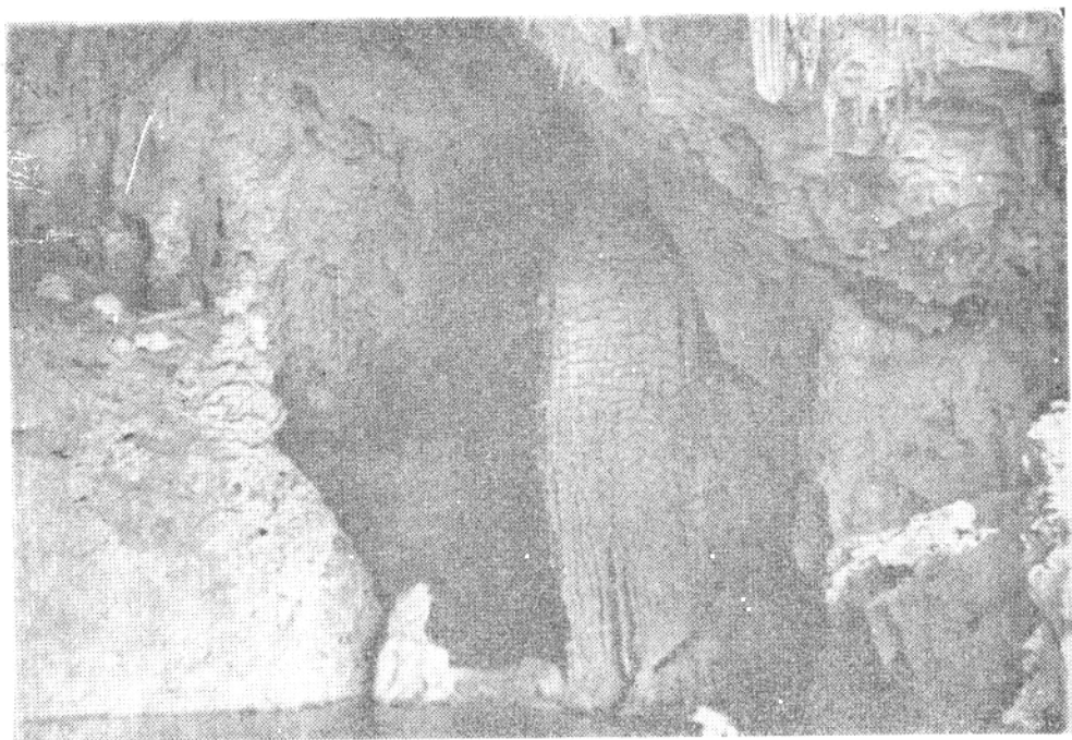
上林县大龙洞水库坝首溢洪洞
