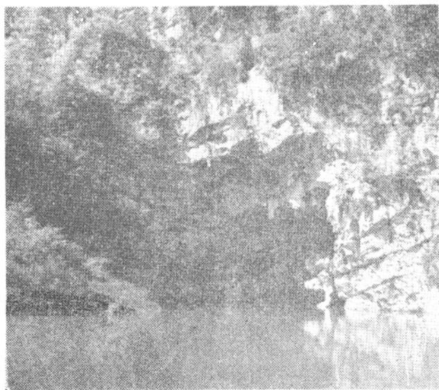
天等县小山地下河出口
