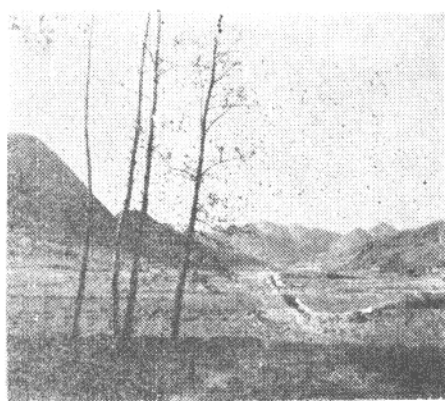
隆林县蛇场公社干坝谷地
