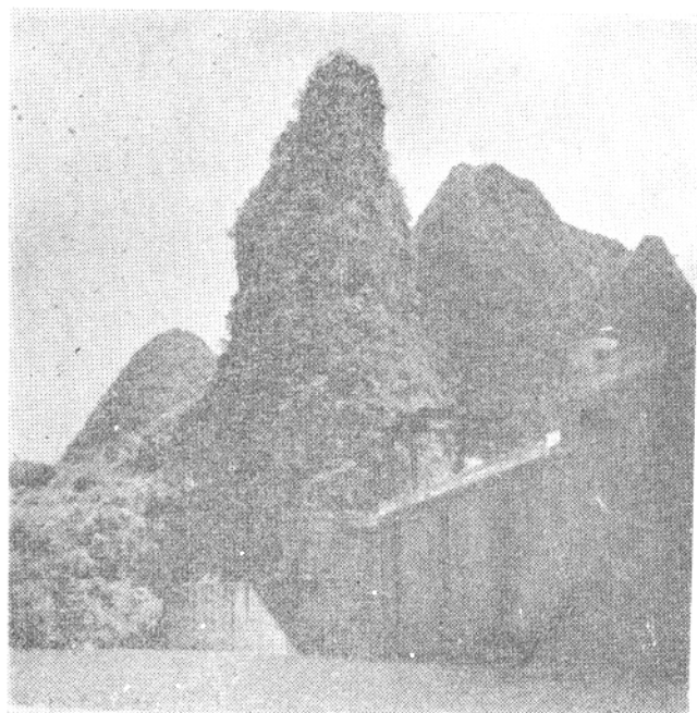
大新县那岸水电站坝址左岸峰林
