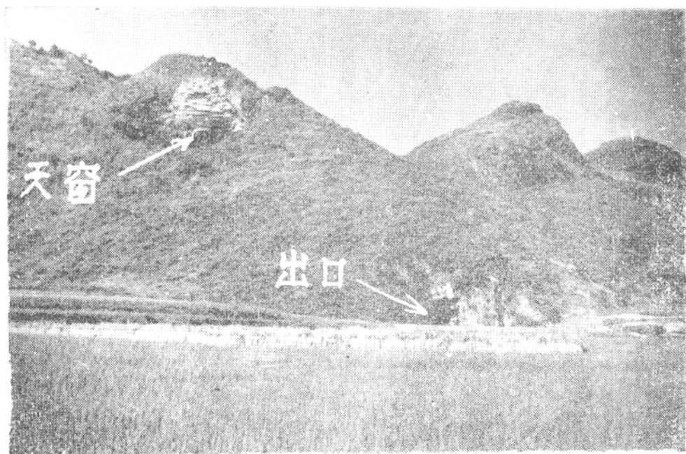
天等县小山地下河出口及天窗全景
