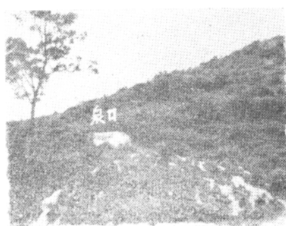
隆林县蛇场公社一上升泉
