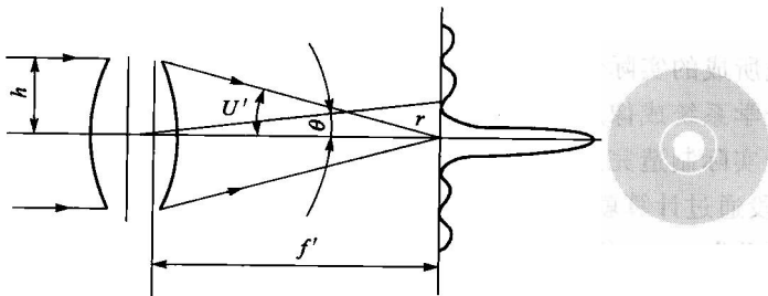
图 1-7 夫朗和斐圆孔衍射图
