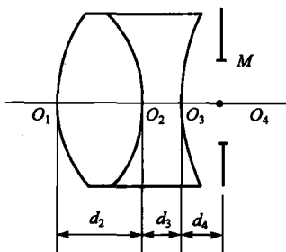
图 1-1 光学系统图
