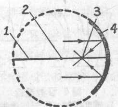
圖3 凹面反光鏡
