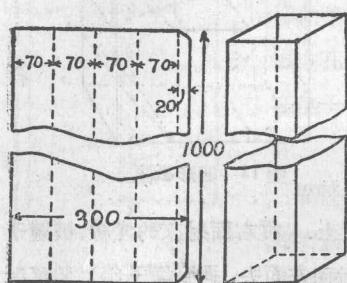
圖 14 長方筒
