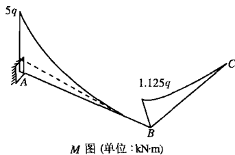
M 图 (单位: \text{kN} \cdot \text{m} )
