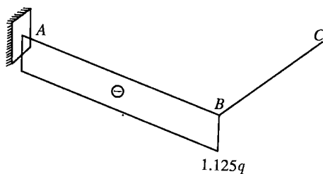
M_i 图(单位: \text{kN}\cdot\text{m} )
