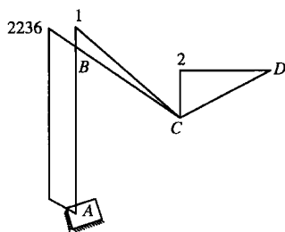
M 图(单位: \text{kN}\cdot\text{m} )
