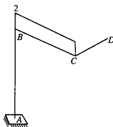
F_Q 图 (单位: kN·m)
