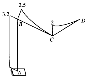
M 图 (单位: kN·m)
