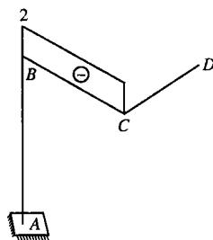
M_i 图(单位: \text{kN}\cdot\text{m} )
