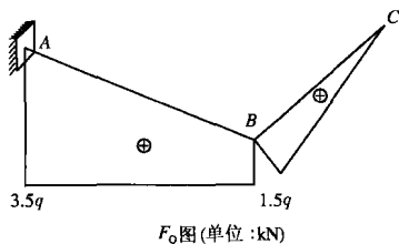
F_Q 图 (单位: \text{kN} )
