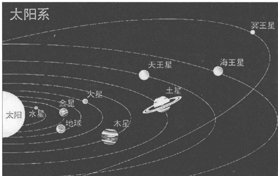
太阳系八大行星及冥王星示意图
