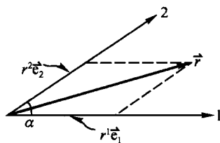
图 1.2 在斜交坐标中, 矢量 \vec{r} 的各分量, 单位矢分别为 \vec{e}_1, \vec{e}_2
