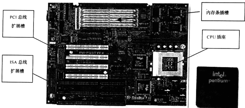
图 1.1.2 主板示意图
