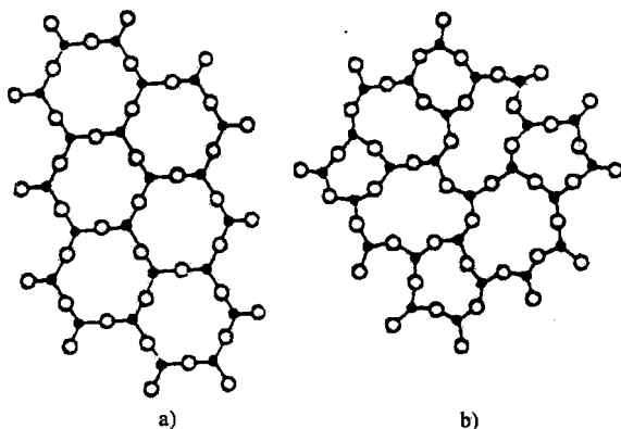
图 11-1 晶体、玻璃体的原子排列示意图 a)晶体;b)玻璃体
