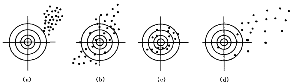
图 1.1.1 测量结果精确度与射击打靶的类比
