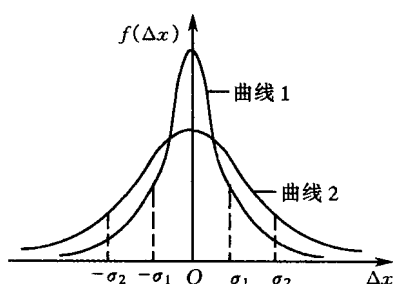
图 1.1.4 \sigma_2 > \sigma_1 的情形
