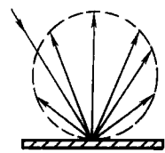
图 1-8 各向同性漫反射
