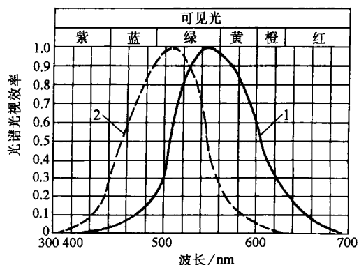
图 1-2 光谱光视效率曲线
