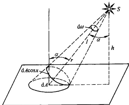
图 1-3 点光源的发光强度
