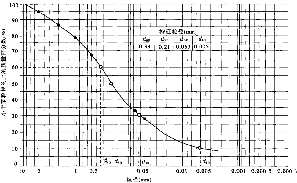
图 1-2 土的颗粒级配曲线
