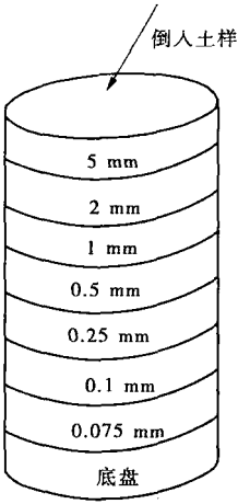
图 1-1 标准筛示意
