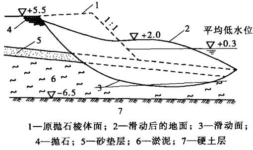
图 0-2 连云港钢板桩码头抛石棱体滑动示意
