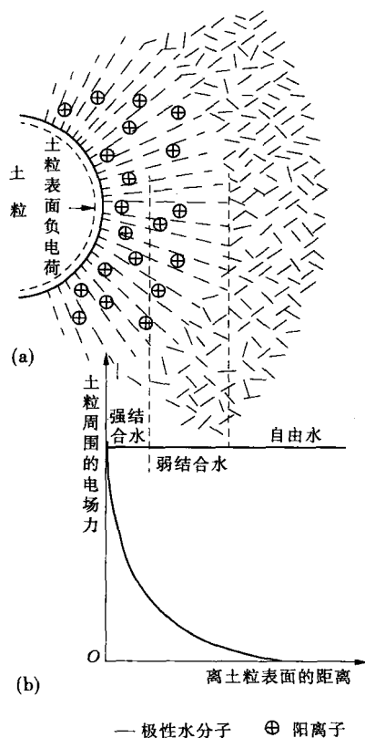
图 1-4 土粒与水分子相互作用的模拟
