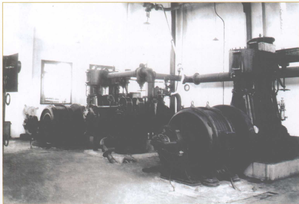
1941年 5月 运抵贵阳，安装于水口寺贵阳电厂的520千瓦发电设备
