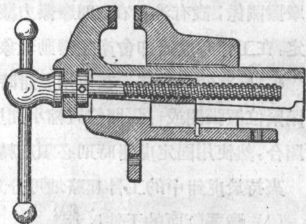
圖 4. 虎鉗構造圖
