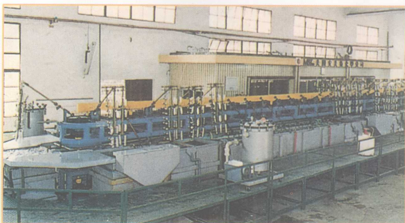
自贡通明电筒灯具 总厂从美国引进的 3 号 光镍铬电镀生产线
