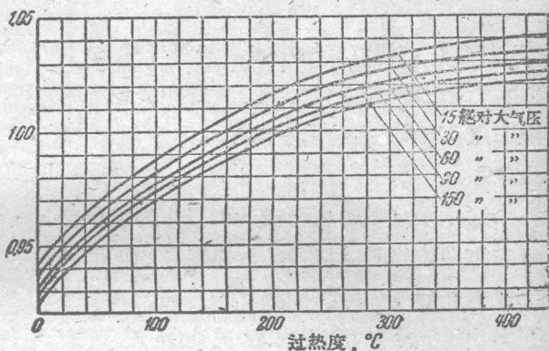
图 7-3. 内效率的修正系数。
