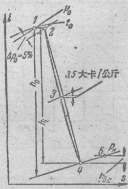
图 7-4. h-s 图上的透平工作过程的作法 (适用于没有中间再热的透平)。
