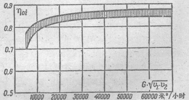
图7-8. 冲动式透平级组的相对內效率与蒸汽的平均容积流量之间的关系。
