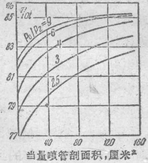
图 7-5. 不同相对压力 p_0/p_2 下(初压对终压之比),具有中间再热的大功率透平以及没有中间再热的双轴透平的高压部分的内效率。
