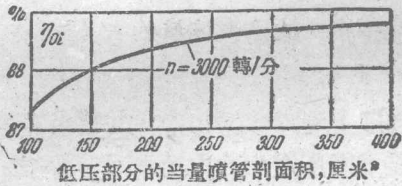
图7-7. 具有中間再热的大型凝汽式透平 低压部分的內效率 \eta_{oi} 。
