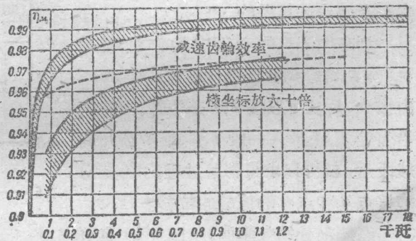
图 7-9. 透平的机械效率曲线以及减速齿轮的机械效率曲线。
