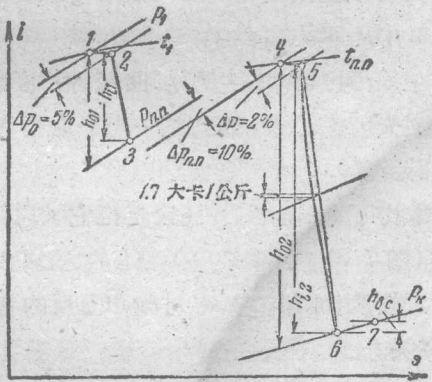
图 7-6. 中间再热式透平中蒸汽膨胀过程在 h-s 图上的作法。
