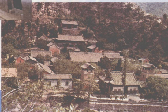
交城玄中寺
