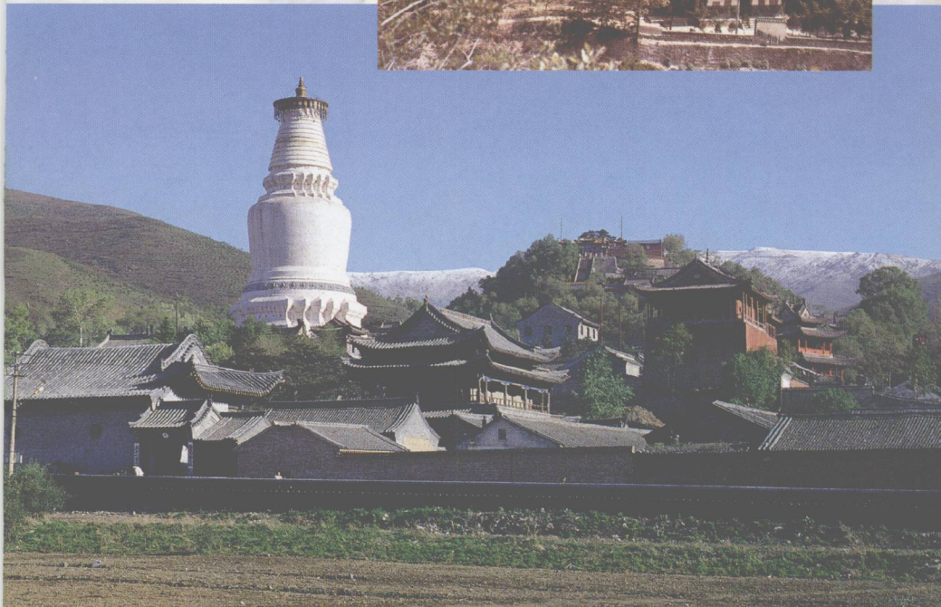
五台山
