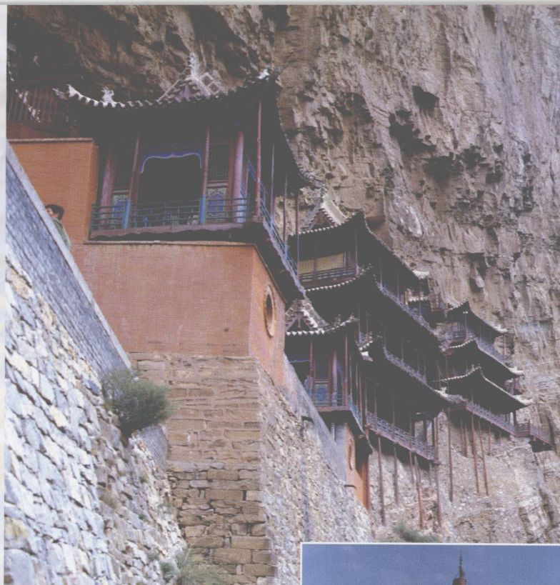
恒山悬空寺
