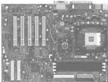
图 1-7 主板
