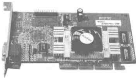
图 1-9 显卡
