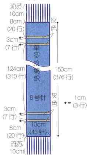
结构图 D
