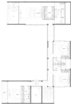
二层平面图
