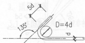
(a) 末端带135°弯钩
