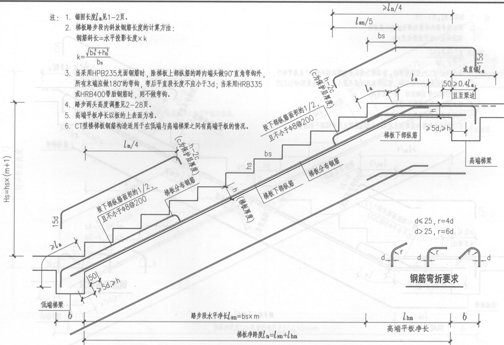
CT型楼梯梯板钢筋构造
