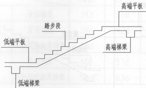
梯板高端单边支座 (楼梯间内的梯梁)
