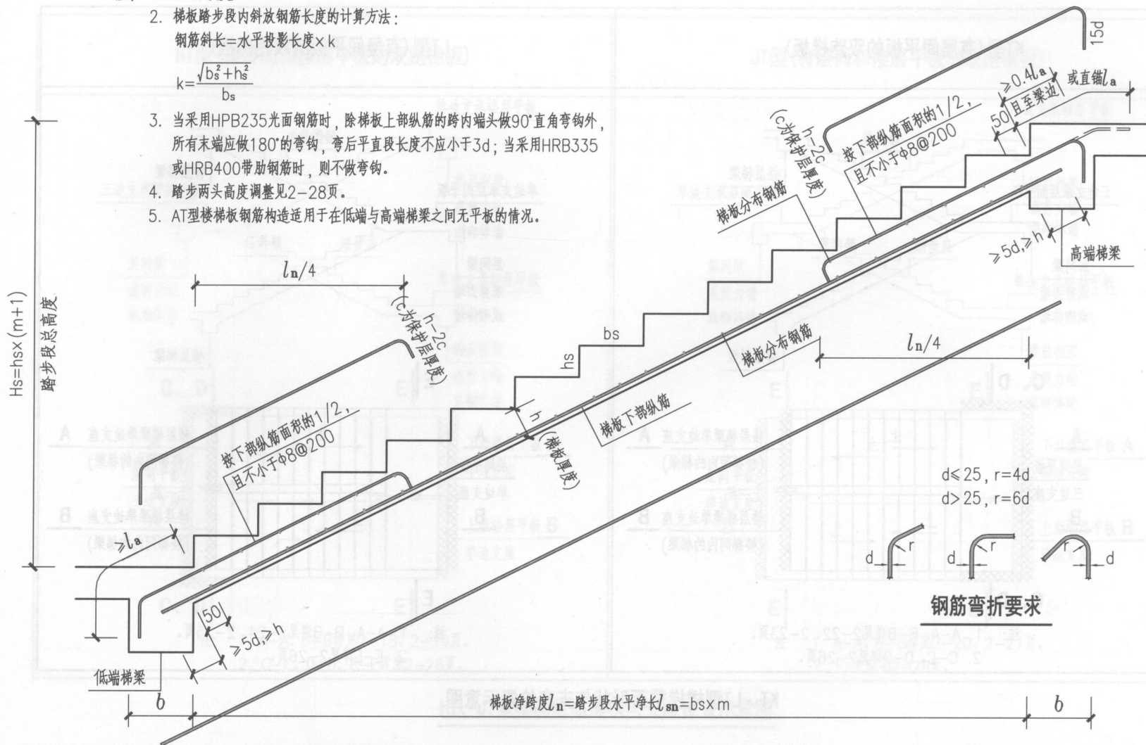
AT型楼梯梯板钢筋构造
