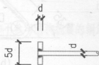
(b) 末端与钢板穿孔塞焊
