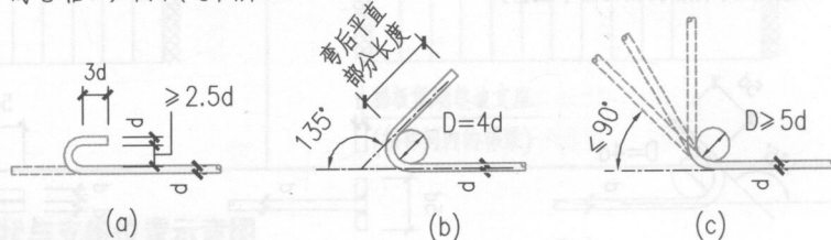
图1 钢筋的弯钩和弯折
