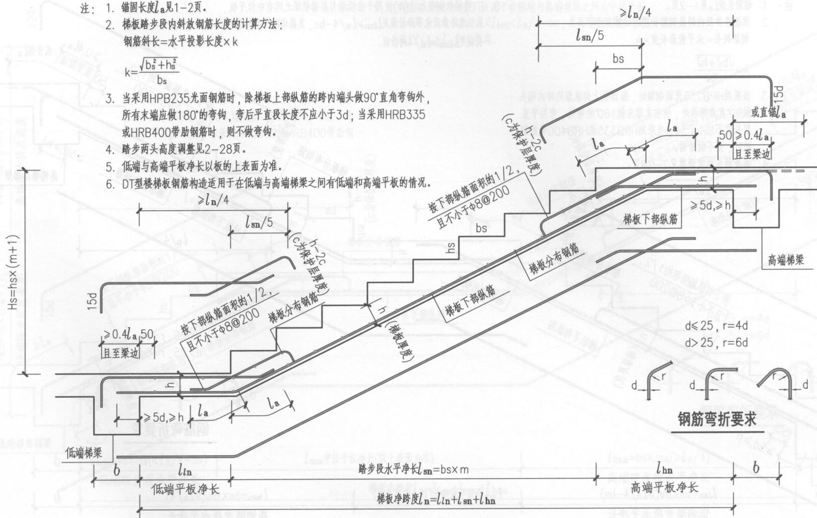
DT型楼梯梯板钢筋构造
