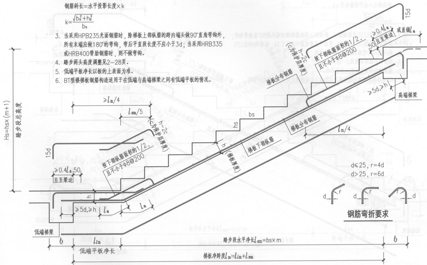
BT型楼梯梯板钢筋构造
