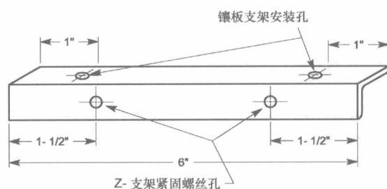
图 1-8 Z-支架元件片。
