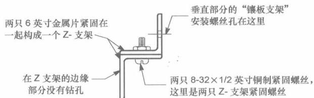
图 1-9 装配 Z-支架。
