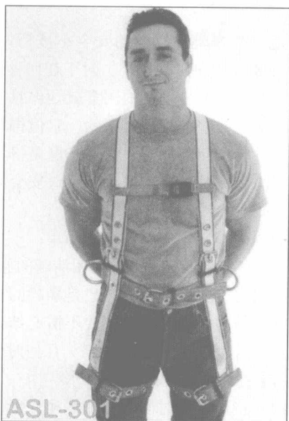
图1-2 垂直保护安全带与攀塔的定位安全带相结合。(图片由Champion Radio Products提供)
