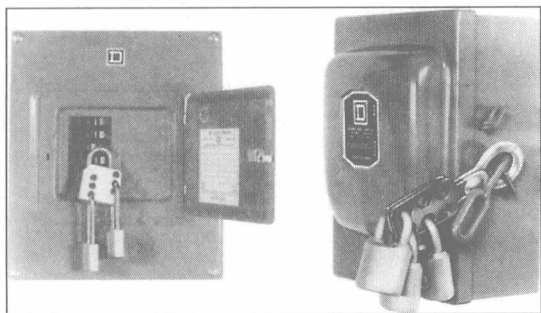
图 1-6 在爬天线塔之前，应把天线开关及电源开关切断，并在盒上加锁并加挂警示牌“严禁合闸”。
