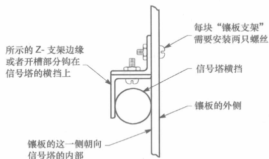
图 1-10 天线塔梯的横挡上安装屏蔽装置。
