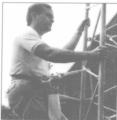
图1-7 Mark Wilson, K1RO示范了系上安全钩的正确方式，将安全钩打开并且正面远离天线塔。通过这种方式连接安全钩就不会因为压在天线塔支架上面而造成意外打开的情况了。
