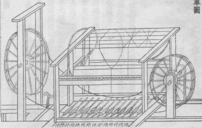
大紡車圖考
