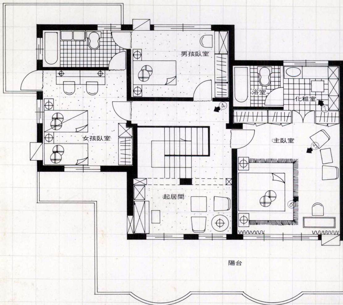
二樓平面圖 1:100cm
