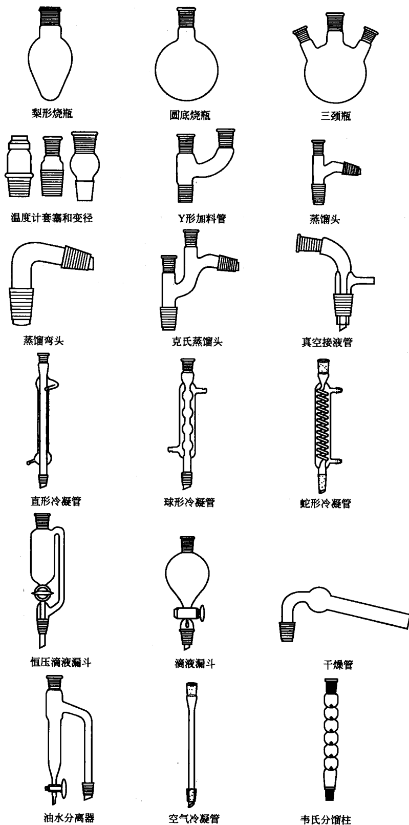
图 1-1 常用标准口玻璃仪器
