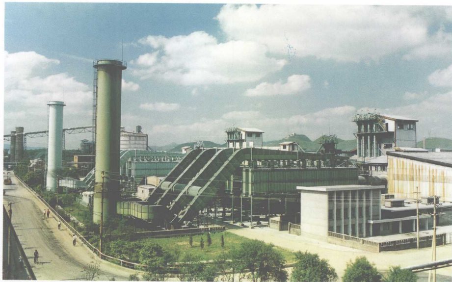
贵州铝厂电解铝生产干法净化系统
