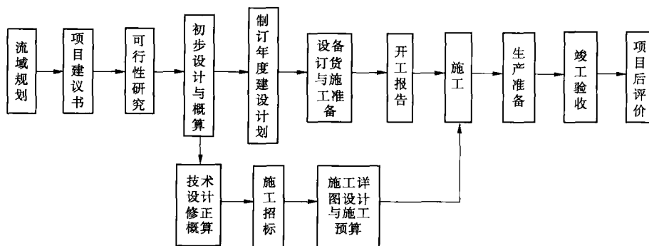
图 1-1 水利工程基本建设程序
