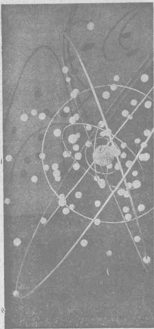
鈾的原子，大圓點是原子核，許多小圓點是電子。
