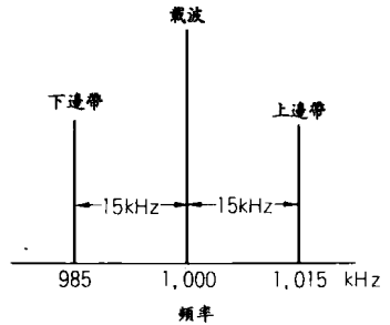
圖 1 - 4 用 15kHz 的信號對 1,000kHz 的載波進行 AM 調制時的頻譜
