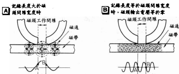
圖 1-2 磁頭工作間隙的寬度必須小於信號最高記錄波長之一週
