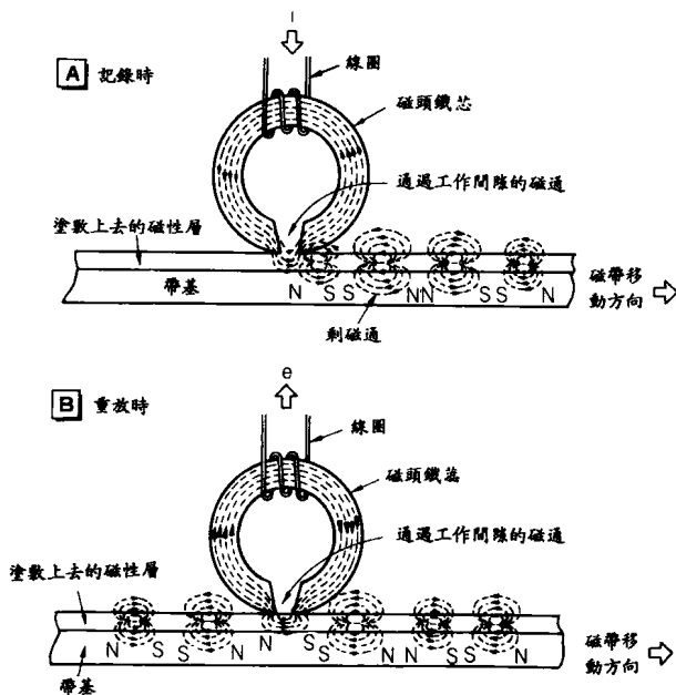
圖 1 - 1 磁頭錄放模式圖
